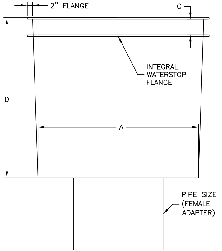
ELEVATION
