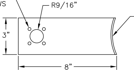
ANEMOMETER MOUNT SCALE: N.T.S.
